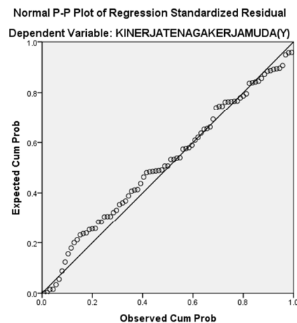
Gambar 3. Uji Normalitas dengan Normal P-Plot Regression Standardized
