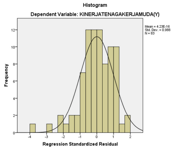
Gambar 2. Uji Normalitas Dengan Histogram
