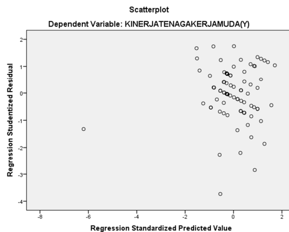
Gambar 4. Uji Heteroskedastisitas Menggunakan Metode Analisis Grafik
